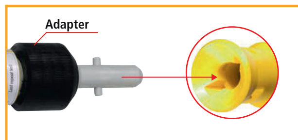
Fig. 2 Isolierstange Spindel-Querstift
